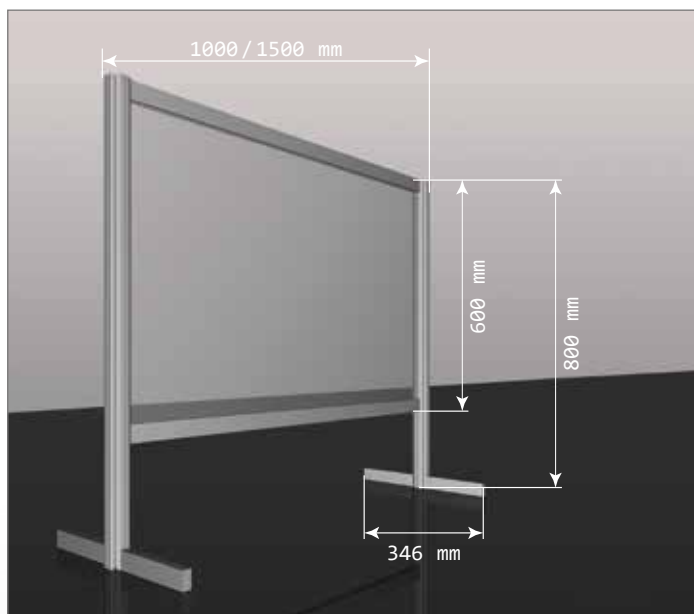
Kontakt-Schutzwand 1000 mm oder 1500 mm
